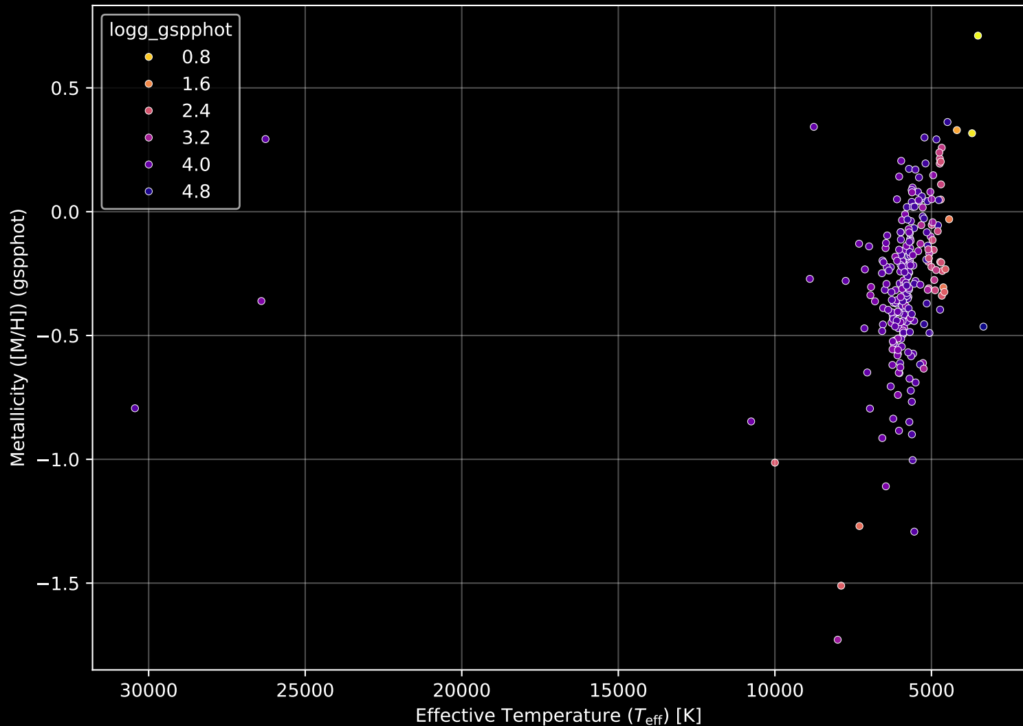
GALAH DR4 Field: [7134] Stellar Population Parameters (n= 247)
