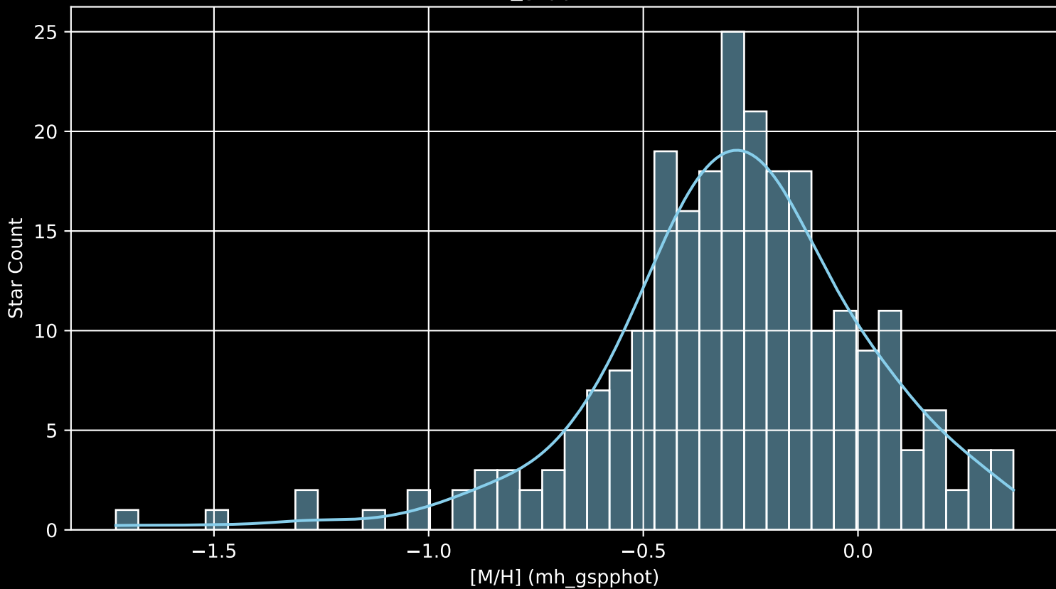
GALAH DR4 Field: [7134] [M/H] (mh_gspphot) (n= 246)
