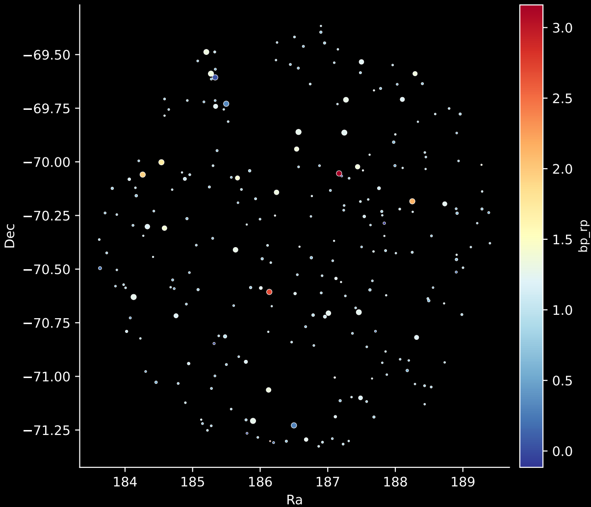
GALAH DR4 Field: [7134] Stars: 247
